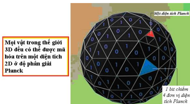
Figure 4 Vũ trụ (Binary Information) 4 diện tích Planck
