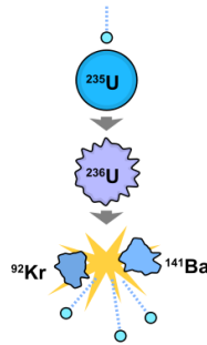
Figure 2 Biểu đồ phản ứng phân hạch Uranium 235
